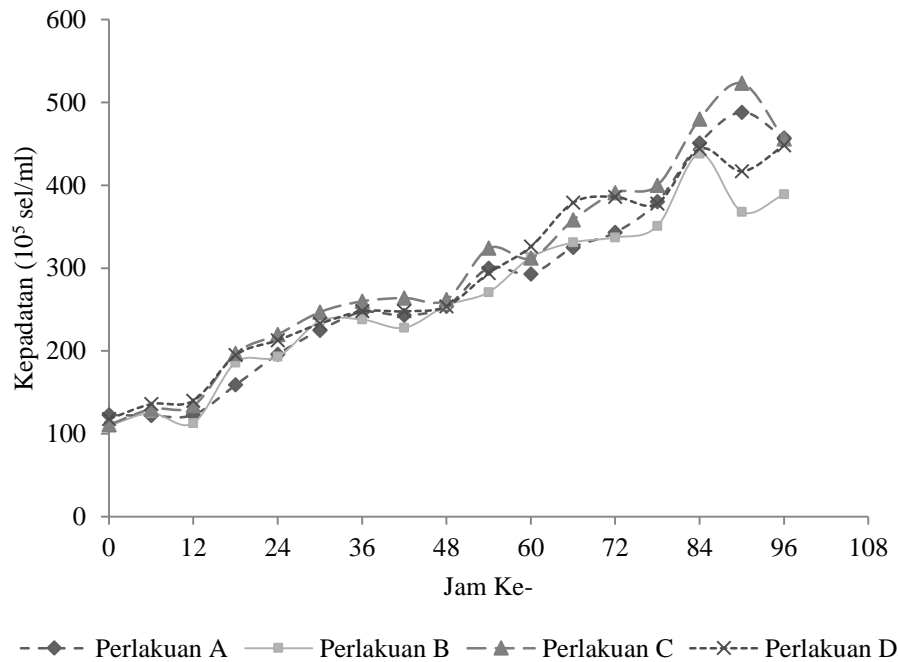
Gambar 2. Kurva pertumbuhan Nannochloropsis sp. pada tiap perlakuan.
