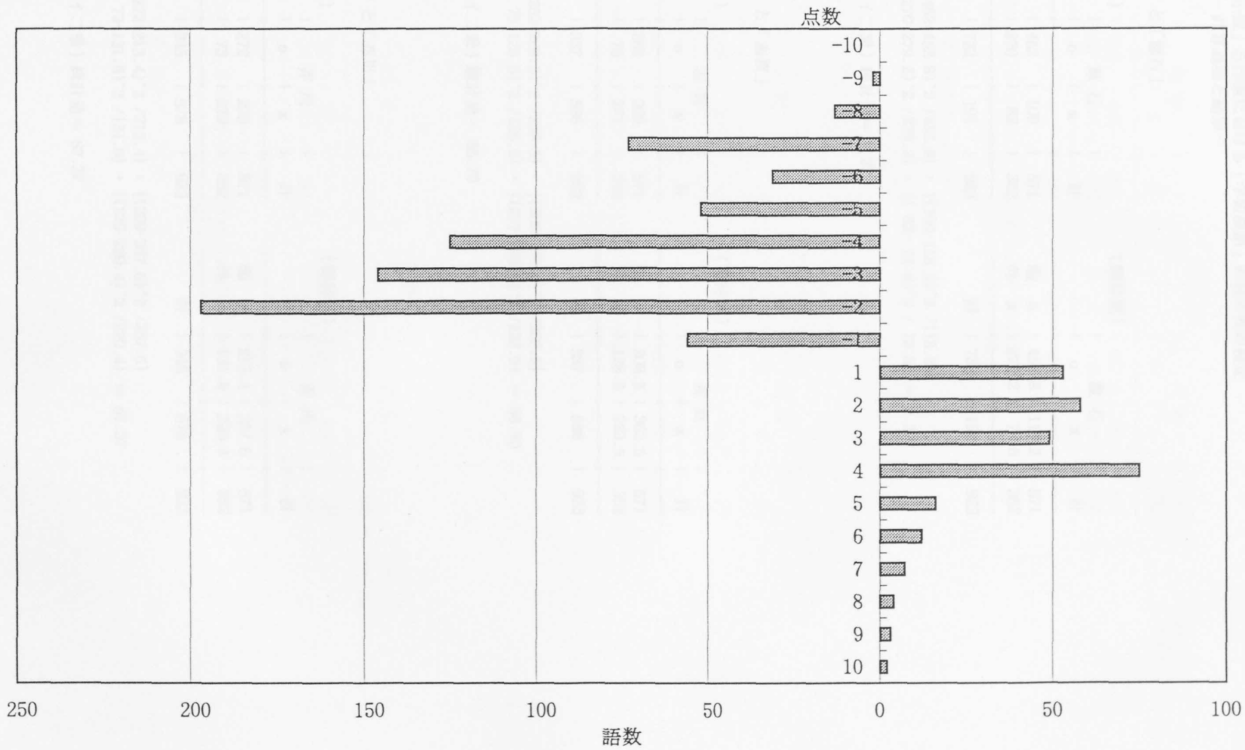
図4.26. 「小説」増加と減少の傾向の語数分布
