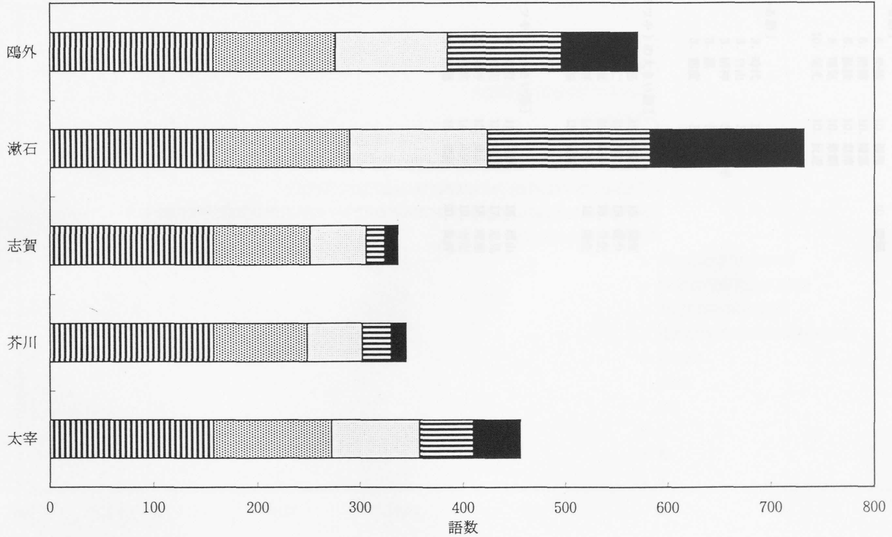
図4.24. 「小説」各作家の共通語数
