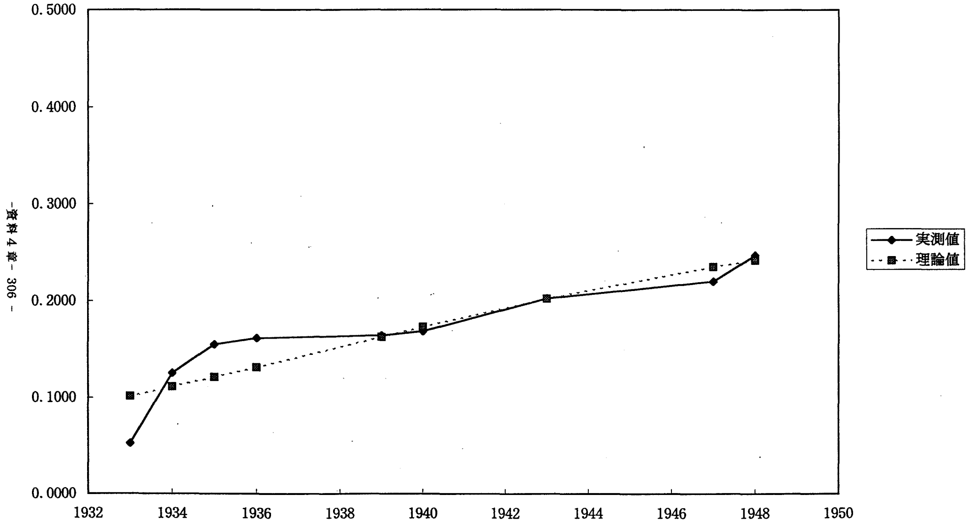
図4.33. 「太宰」データと Piotrowskiカーブの比較
