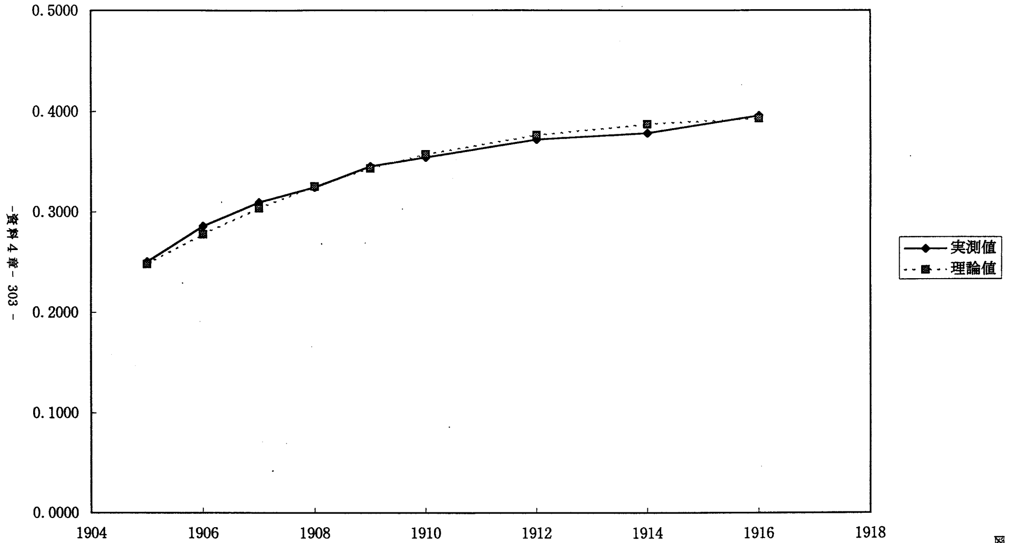
図4.30. 「湫石」データと Piotrowskiカーブの比較
