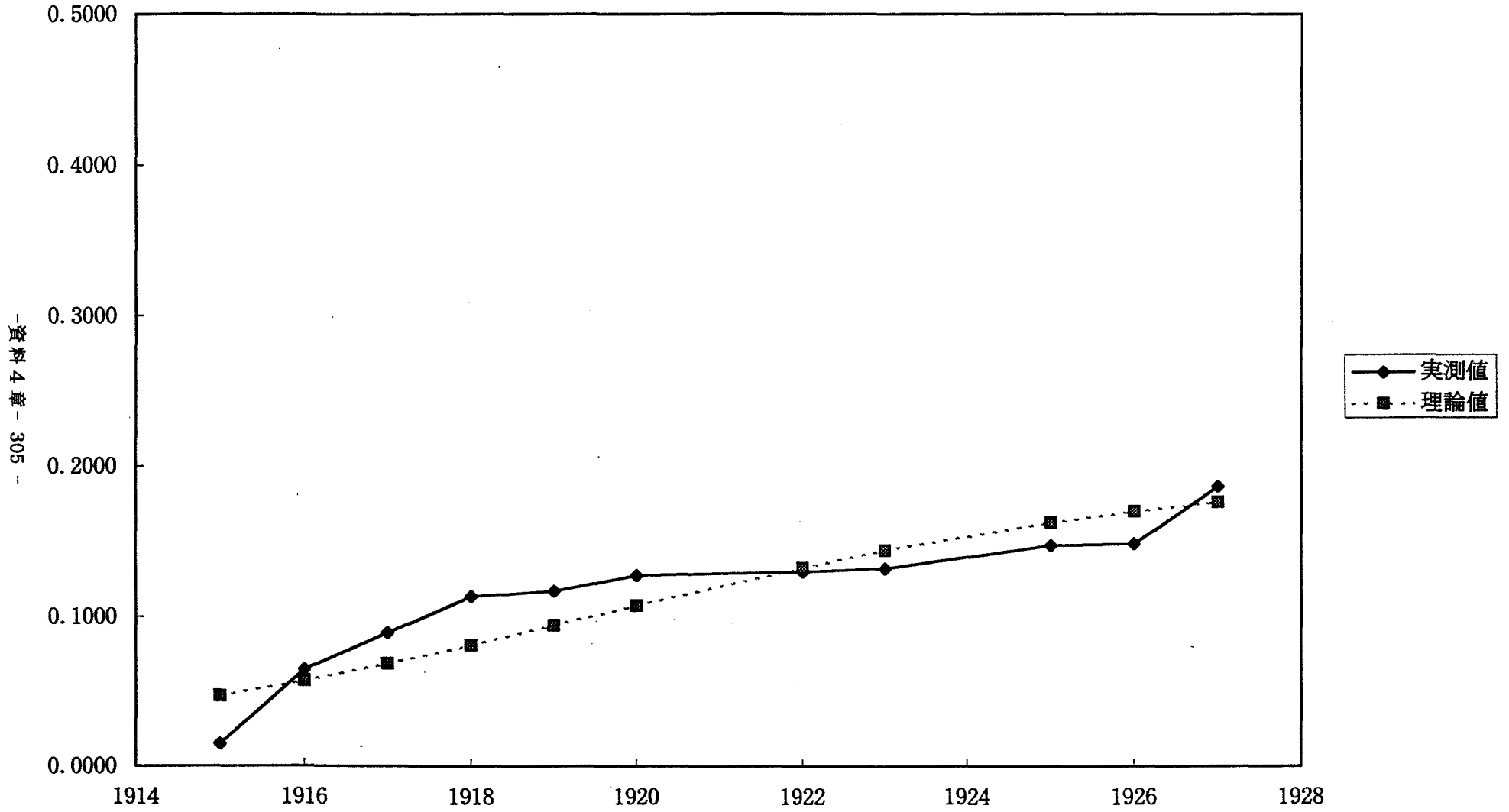
図4.32. 「芥川」データと Piotrowskiカーブの比較
