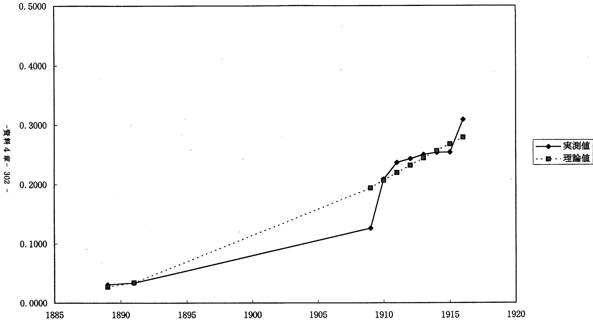
図4.29. 「鷗外」データと Piotrowskiカーブの比較
