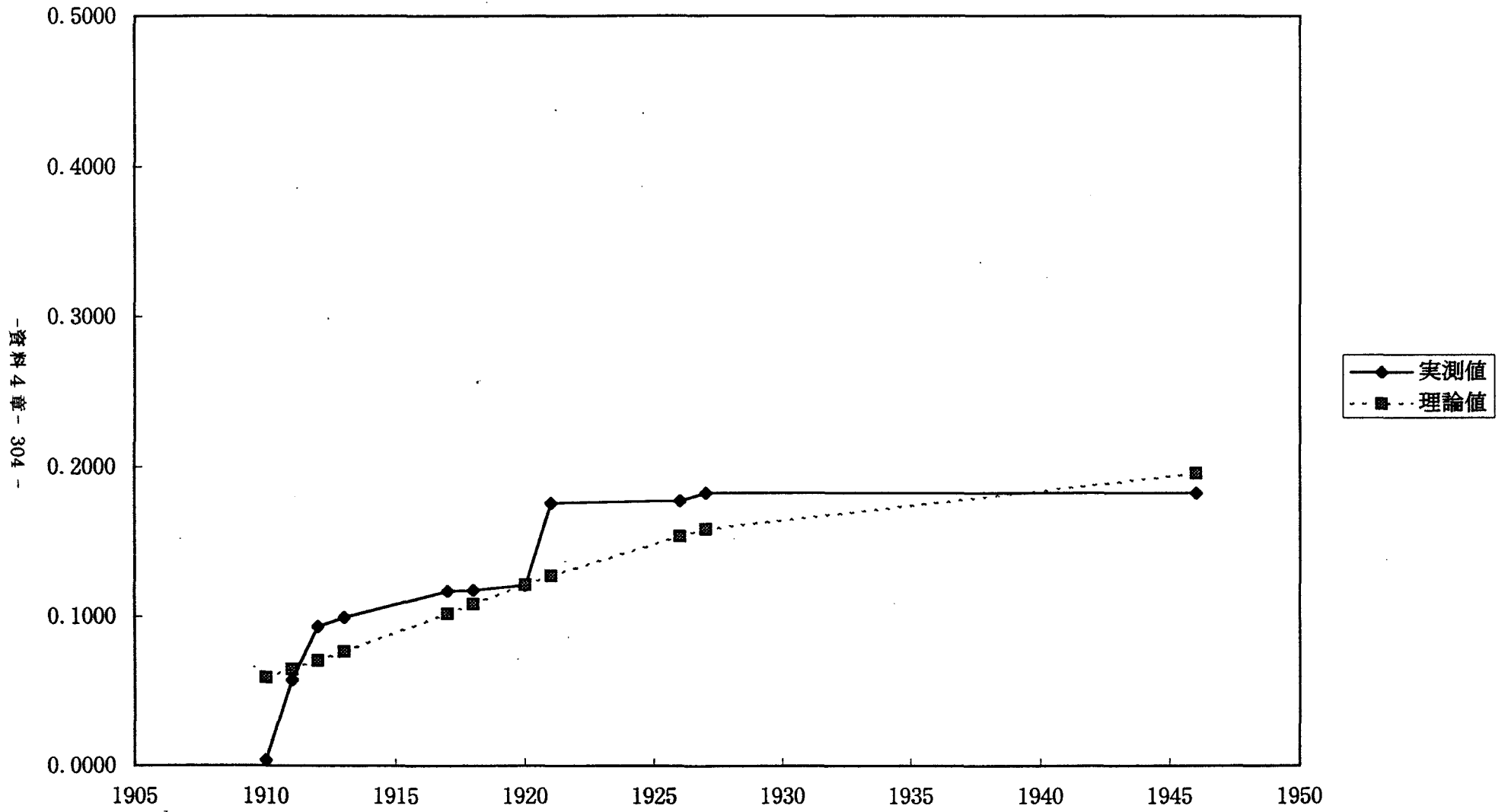
図4.31. 「志賀」データと Piotrowskiカーブの比較
