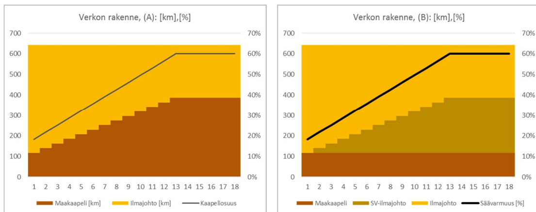
Kuva 12. Verkon rakenne, kun sovelletaan strategiaa A (vasen) ja strategiaa B (oikea). SV-ilmajohhto tarkoittaa säävarmaa ilmajohtoa, joka on toteutettu lokaalein toimenpitein. Toimintaohjelma muodostuu kaapeliosuuden/säävarman verkon osuuden kasvattamisesta 18 %:sta 60 %:iin 12 vuodessa.
