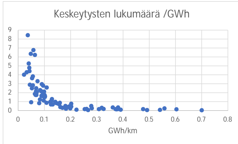
Kuva 27. Keskeytysten lukumäärän ja jakelun energiatiheiden välinen riippuvuus.
