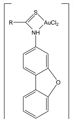
11a R=Me 11b R=Ph 11c R=2-furyl
