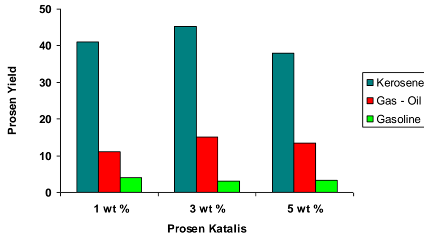
Gambar 2. Yield biofuel dari reaksi hydrocracking minyak sawit dengan variasi jumlah katalis dalam prosen berat (wt. %)
