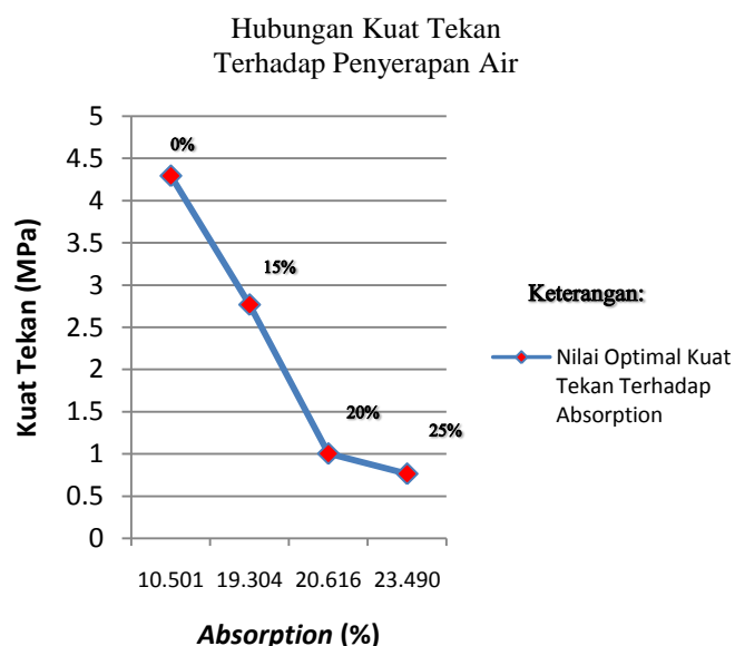
Gambar 7. Hubungan Kuat Tekan Terhadap Penyerapan Air Lockbrick Moduler
