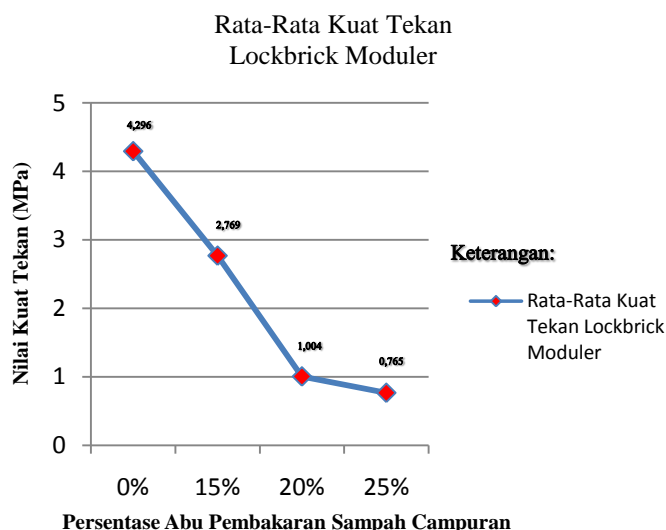
Gambar 5. Nilai Rata-Rata Kuat Tekan Lockbrick Moduler
