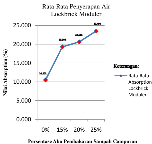
Gambar 6. Nilai Rata-Rata Penyerapan Air Lockbrick Moduler
