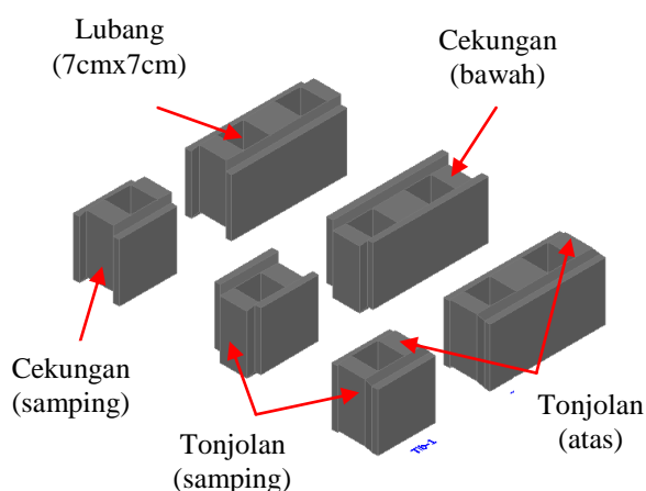
Gambar 2. Produk Lockbrick Moduler (Sumber: Habsya, 2005)
