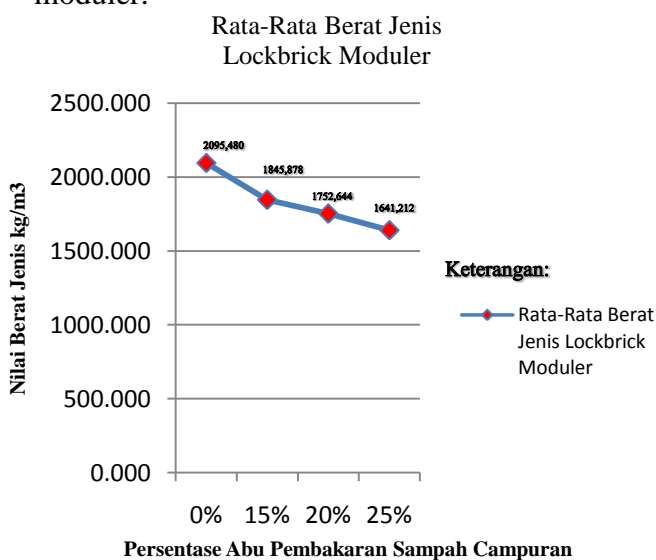
Gambar 4. Nilai Rata-Rata Berat Jenis Lockbrick Moduler
