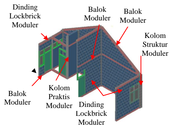
Gambar 1. Potongan 3D Rumah Tumbuh (Sumber: Habsya, 2005)
