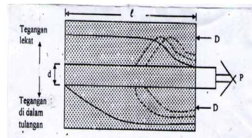
Gambar 2 Percobaan Kekuatan Lekat (Sumber : Y. Soehardono, 1989: 58)
