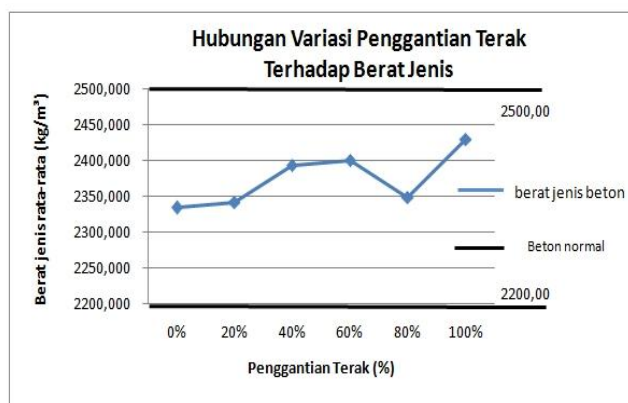
Gambar 4 Hasil Pengujian Berat Jenis
