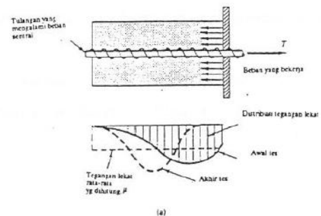
Gambar 1 Percobaan pencabutan (Nawy, 1990 : 399.)
