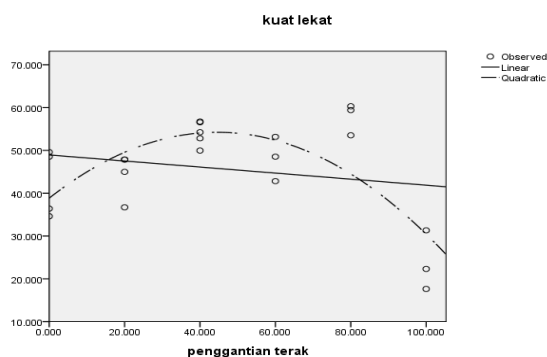
Gambar 3 Hasil Pengujian Kuat Lekat
