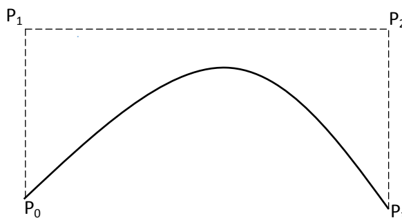
Gambar 2. Empat Titik Bézier Curve
