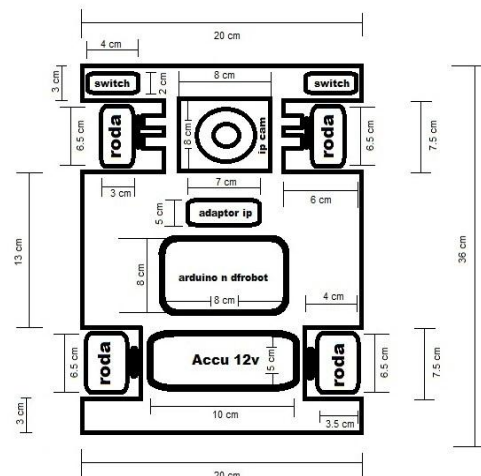
Gambar 4. Rancangan Mobil Kontrol
