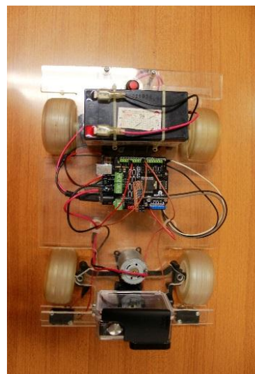
Gambar 6. Rangka Mobil Tampak atas
