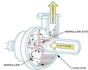
Gambar 3. Pompa Sentrifugal (Sularso, 2006)
