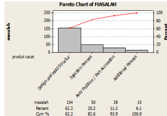
Gambar 2. Diagram Pareto Penyebab Kerusakan Mold .
