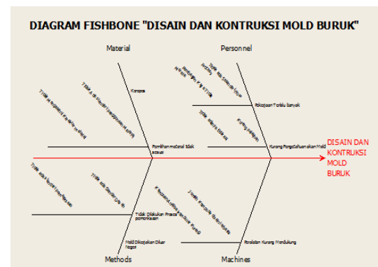
Gambar 3. Fishbone Diagram "Desain dan Kontruksi Mold Buruk"
