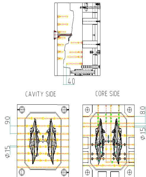
Gambar 11. Desain Saluran Pendingin
