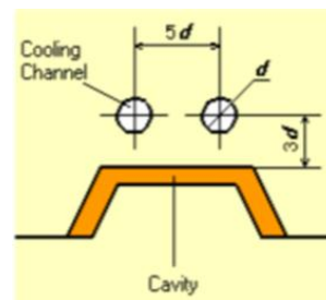
Gambar 6. Standar Jarak Lubang Pendinginan.
