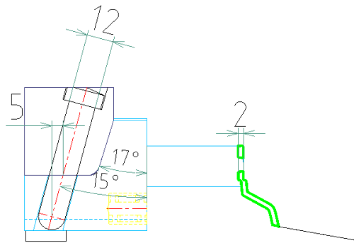
Gambar 12. Desain Slider
