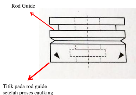
Gambar 1. Rod Guide
