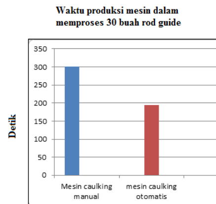
Gambar 6. Grafik perbandingan cycle time mesin caulking manual dengan mesin caulking otomatis
