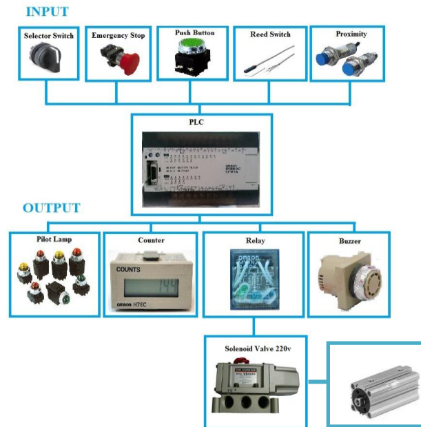
Gambar 3. Rancangan sistem kontrol mesin caulking rod guide otomatis
