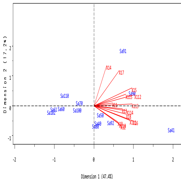
Gambar 1 – Analisis Biplot peubah X1 Sangihe
