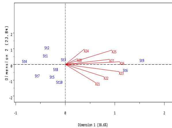
Gambar 6 – Analisis Biplot peubah X2 Sitaro
