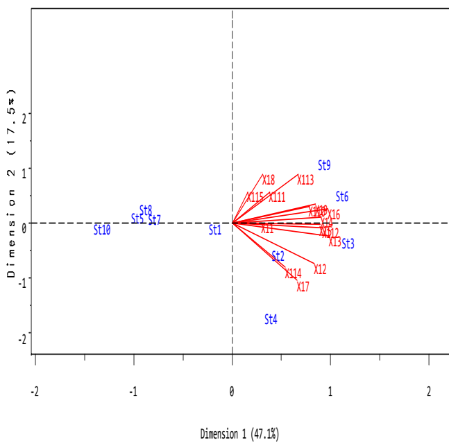
Gambar 5 – Analisis Biplot peubah X1 Sitaro
