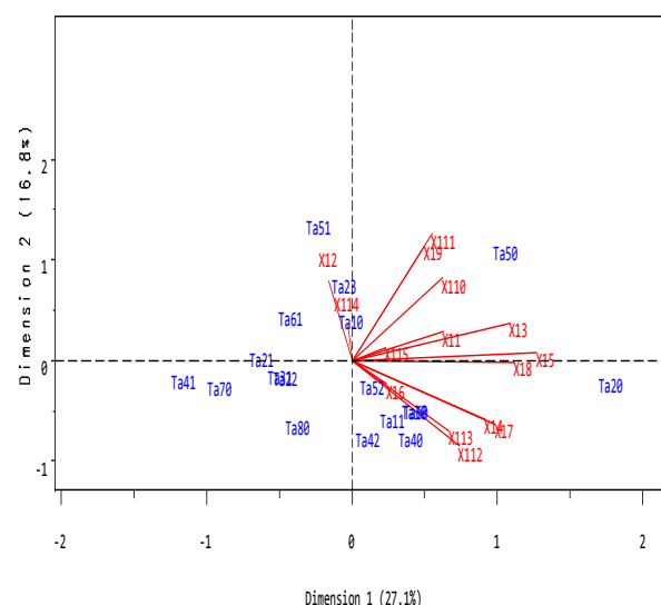
Gambar 3 – Analisis Biplot Peubah X1 Talaud
