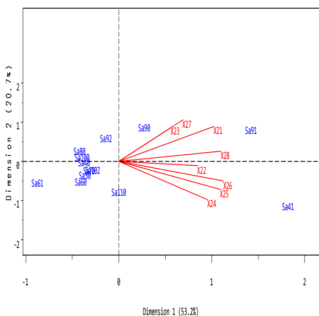
Gambar 2 – Analisis Biplot peubah X2 Sangihe
