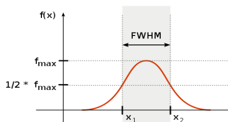
Gambar 1. Difaktogram FWHM
