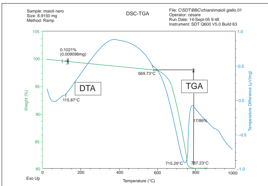
Figura 31. Analisi termica della porzione di intonaco del campione nero.
