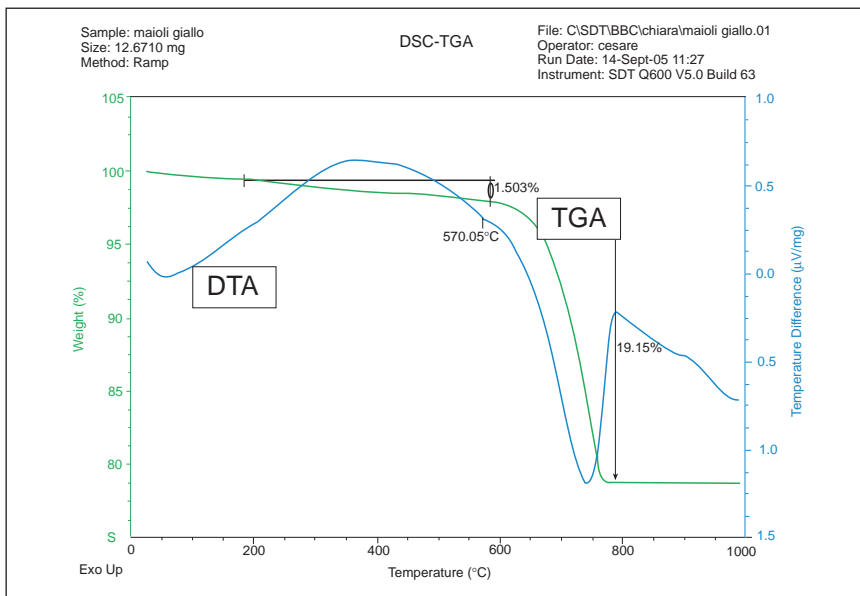
Figura 30. Analisi termica della porzione di intonaco del campione giallo.
