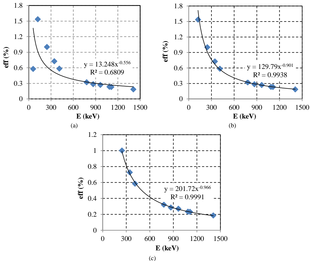
Gambar 3. Perbandingan kurva efisiensi terhadap energi dengan menggunakan energi mulai 59,5 keV (a), energi mulai 121,8 keV, (b), dan energi mulai 244,7keV, (c) pada jarak sumber-detektor 5 cm
