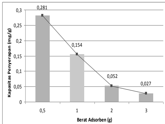
Gambar 2 Perbandingan Kapasitas Penyerapan Logam Cr untuk Variasi Berat Adsorben
