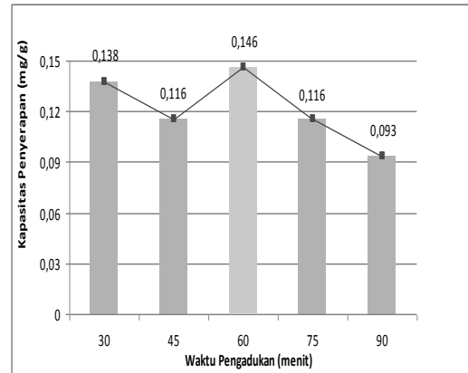
Gambar 5 Perbandingan Kapasitas Penyerapan Logam Cr untuk Variasi Waktu Kontak
