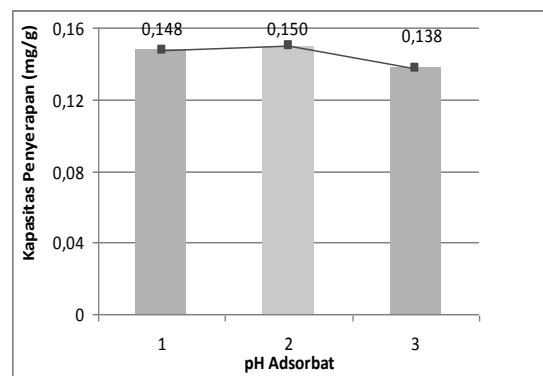
Gambar 3 Perbandingan Kapasitas Penyerapan Logam Cr untuk Variasi pH Adsorbat
