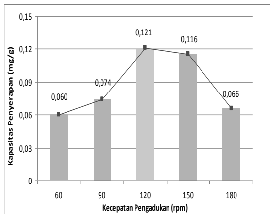
Gambar 4 Perbandingan Kapasitas Penyerapan Logam Cr untuk Variasi Kecepatan Pengadukan
