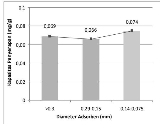
Gambar 1 Perbandingan Kapasitas Penyerapan Logam Cr untuk Variasi Diameter Adsorben
