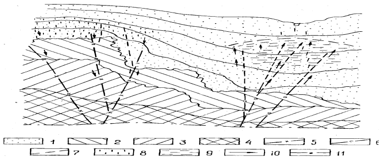
Рис. 6. Схема тектоно-гидравлического механизма гидросферы под влиянием неотектоники (Гаев, 1989): 1 – породы осадочного чехла; 2 – гранитная оболочка земной коры; 3 – базальтовая оболочка земной коры; 4 – верхняя часть мантии с астеносферой; 5 – тектонические нарушения с увеличивающейся скважностью за счет глыбовых поднятий; 6 – тектонические нарушения с уменьшающейся скважностью за счет отрицательных тектонических движений литосферы и верхней мантии; 7 – оперяющая тектоническая трещиноватость; 8 – зоны пьезоминимумов; 9 – гидроаномалии и пьезомаксимумы; 10 – преобладающее направление движения флюидов; 11 – подошва астеносферы как нижняя граница гидросферы, изменяющая свое положение в зависимости от знака тектонических движений
