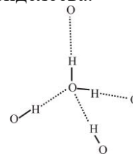
Рис. 3. Тетраэдрическое строение структуры воды и водных растворов, по Дж. Берналу и Р. Фаулеру (1933)
