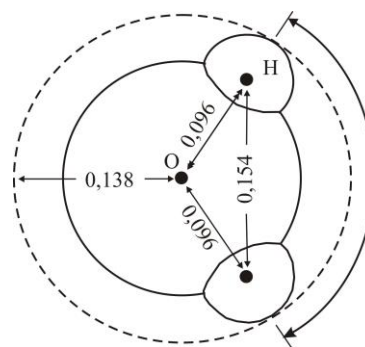
Рис. 5. Гидроль молекулы воды при высокой температуре с плоскими, межатомными связями равнобедренного треугольника и углом при вершине в 104^\circ (межъядерные расстояния даны в нм)
