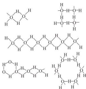
Рис. 4. Кольцевые структуры агрегатов молекул воды пяти конфигураций с водородными мостиками во внешних оболочках Земли, по М. Агено (1967)
