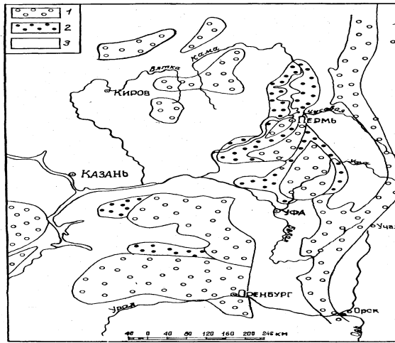
Рис. 7. Схема Приуралья с неоготектоническими поднятиями и очагами дегазации флюидов (Гаев, 1989): 1 – площади с очагами дегазации флюидов, деминерализации рассолов и зонами поглощения; 2 – унаследованные зоны поглощения; 3 – площади, где зоны поглощения не установлены
