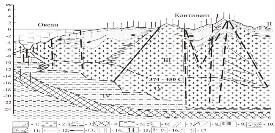
Рис. 2. Модель гидросферы Земли с двумя областями питания и разгрузки вод: 1 – осадочный чехол земной коры и его подошва; 2 – гранитная и базальтовая оболочки земной коры; 3 – верхняя мантия над астеносферой и граница Моховичича; 4 – ювенильная область питания и раз-
