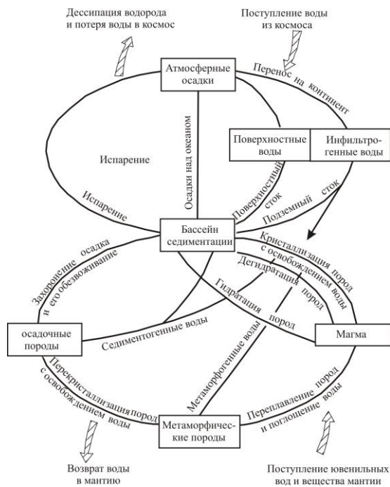
Рис. 1. Взаимосвязь гидрологической и геологической ветвей круговорота воды в земных недрах (Пиннекер, 1984)
