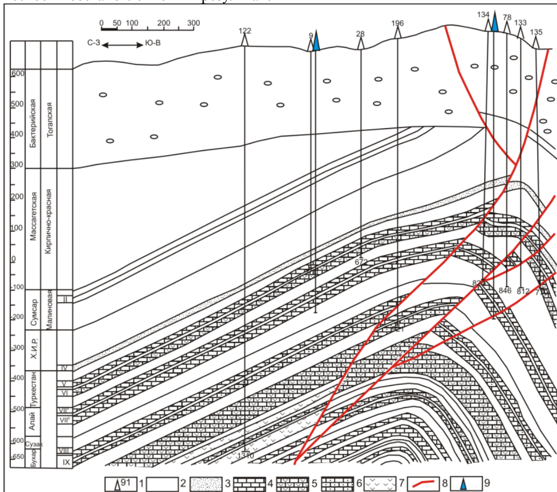
Рис.2. Геологический профиль вкост простирания складки Палванташ по линии V-V: 1 – нефтяные скважины; 2 – глины; 3 – песчаники; 4 – известняки; 5 – ангидриты; 6 – песчаники; 7 – гипсы; 8 – линии нарушений; 9 – проектируемые скважины
