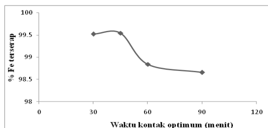
Gambar 2 Kurva hubungan antara waktu kontak optimum (menit) terhadap %Fe terserap
