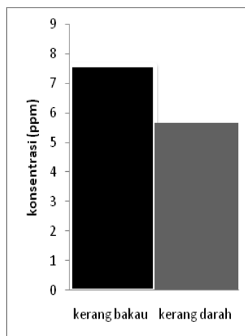
Gambar 1. Data Konsentrasi Logam Timbal Menggunakan Alat Spectro Direct.
