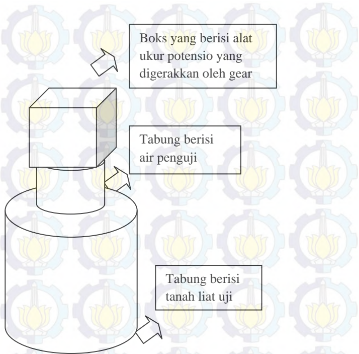
Gambar 3.3 rancang bangun sistem pengukuran dengan metode falling head yang dimodifikasi
