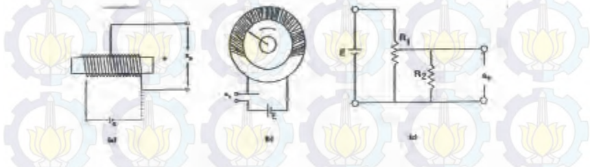
Gambar 2.4 Transduser simpangan potensiometer. (a). Gerakan linier (b). Gerakan sudut (c). Rangkaian. (Mengko, 1988)
