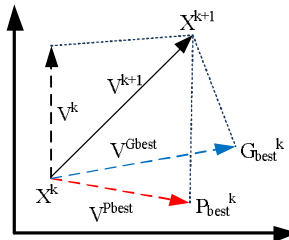
Gambar 3.1 Konsep pencarian P_{best} dan G_{best} dari PSO
