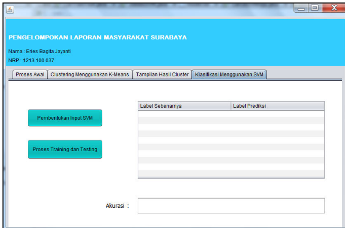
Gambar 4. 12 Tab Klasifikasi menggunakan SVM
