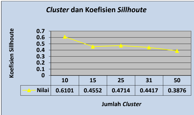
Gambar 5. 1 Grafik Cluster dan Koefisien Sillhouette
