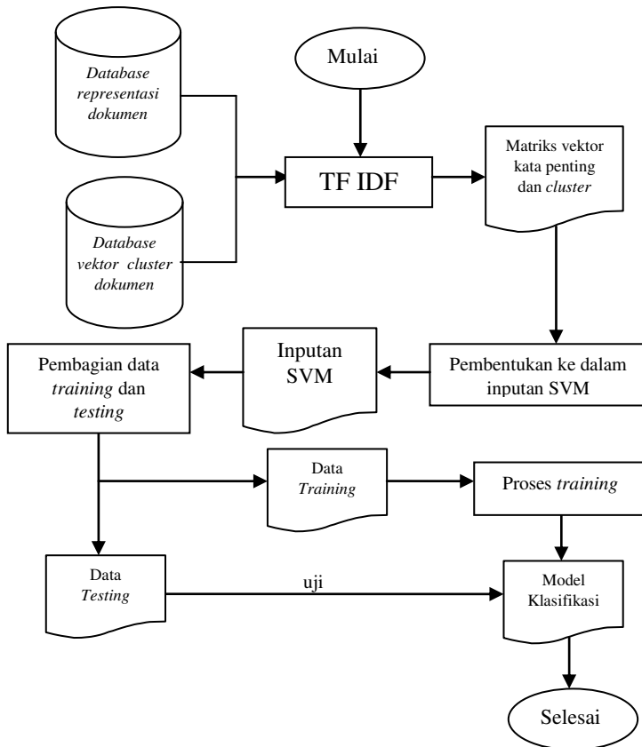
Gambar 4. 7 Diagram Alir Klasifikasi
