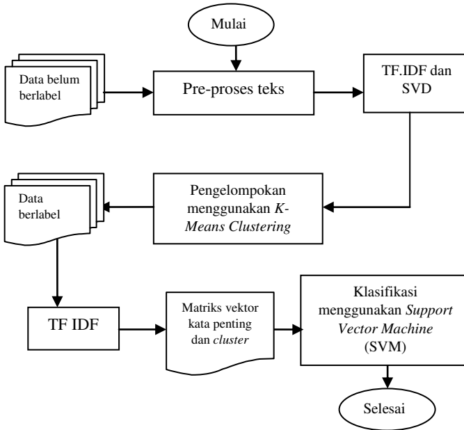
Gambar 4. 1 Diagram Alir Sistem
