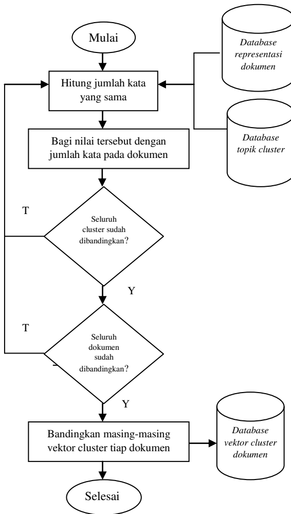
Gambar 4. 6 Diagram Alir Pembentukan Vektor Dokumen
