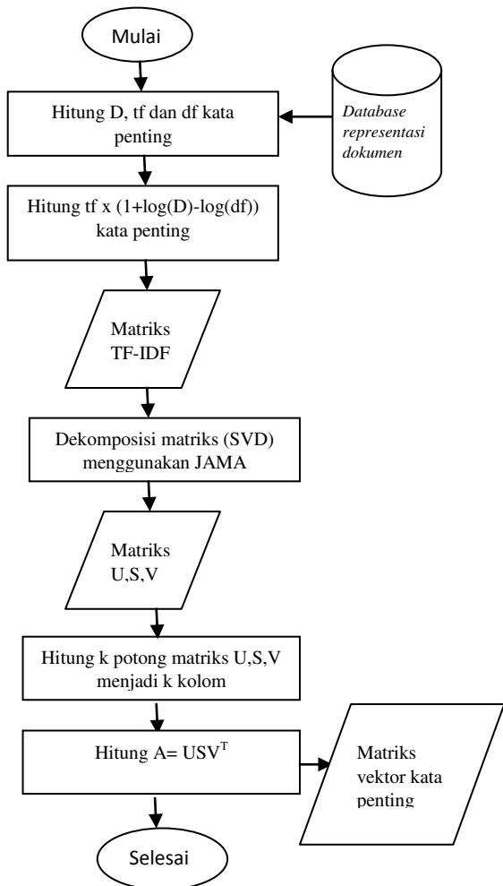
Gambar 4. 4 Diagram Alir Pembobotan
