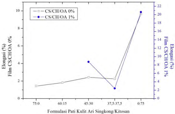
Gambar 4.12 Perbandingan % elongasi Film pada Formulasi CS/CH/OA 0% dan CS/CH/OA 1%
