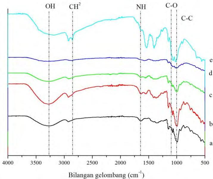
Gambar 4.6 Spektra Inframerah Film Pati Kulit Ari Singkong/Kitosan/Asam Oleat dengan Formulasi (a) CS 75 /OA 0%, (b) CS 60 /CH 15 /OA 0%, (c) CS 45 /CH 30 /OA 0%, (d) CS 37,5 /CH 37,5 /OA 0% dan (e) CH 75 /OA 0%
