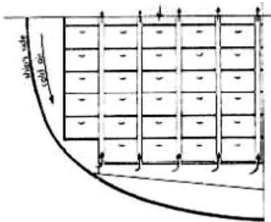
Gambar 2.16. Potongan melintang susunan keranjang ikan dalam palkah
