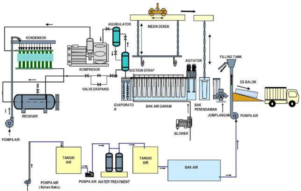
Gambar 2.19 : Proses skema produksi es balok
