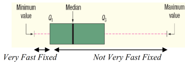
Gambar 2.1 Visualisasi pengkategorian kelas bug 1 (Abdelmoez, 2012)
