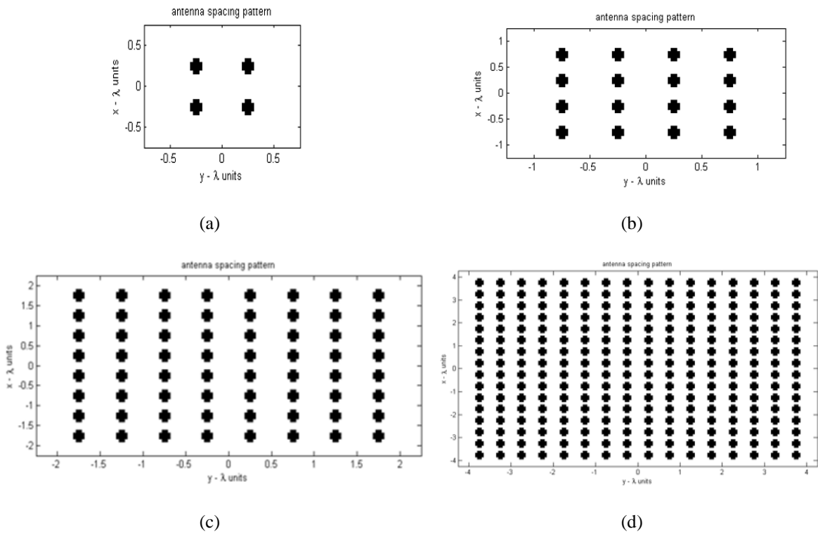
Figure 2. (a) 2x2, (b) 4x4, (c) 8x8, (d) 16x16 planar array arrangement
