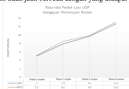
Gambar 9 Grafik perbandingan packet loss data UDP kondisi pemutusan router
