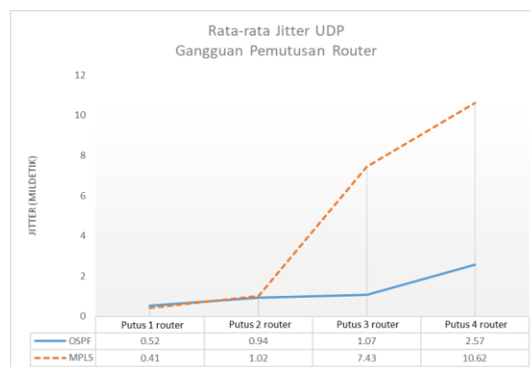
Gambar 8 Grafik perbandingan jitter data UDP kondisi pemutusan router
