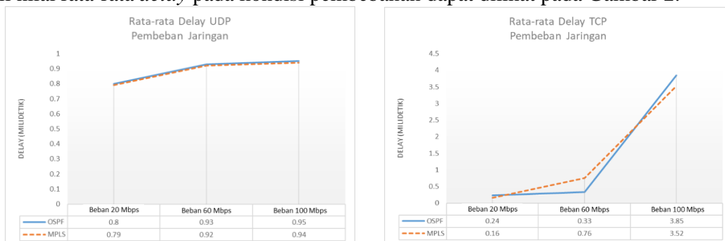
Gambar 2 Grafik perbandingan delay data UDP dan TCP kondisi pembebanan
