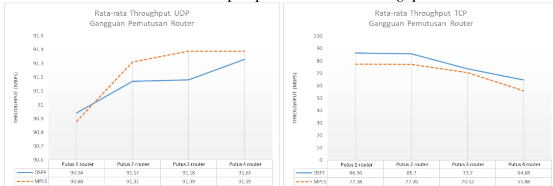
Gambar 7 Grafik perbandingan throughput data UDP dan TCP kondisi pemutusan router
