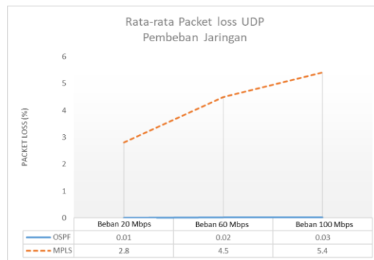
Gambar 5 Grafik perbandingan packet loss data UDP kondisi pembebanan
