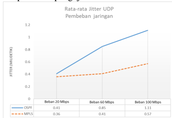
Gambar 4 Grafik perbandingan jitter data UDP kondisi pembebanan
