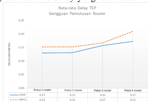
Gambar 6 Grafik perbandingan delay data TCP kondisi pemutusan router
