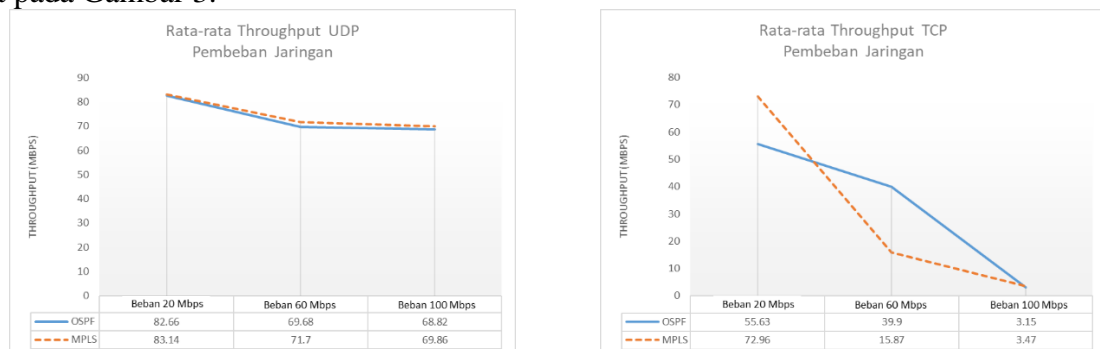
Gambar 3 Grafik perbandingan throughput data UDP dan TCP kondisi pembebanan
