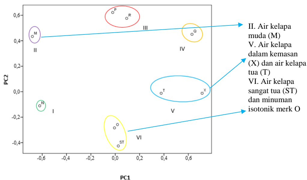
Gambar 4. Hasil PCA berdasarkan data derivatif kedua data absorbansi.
