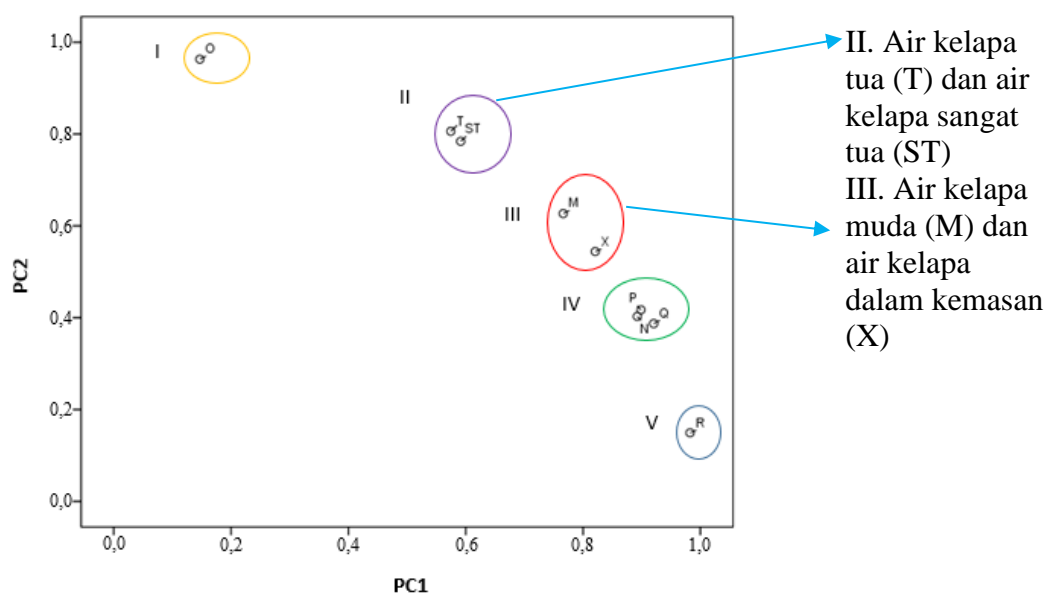
Gambar 2. Hasil PCA dari 9 sampel yang dianalisis menggunakan spektra UV-Vis.
