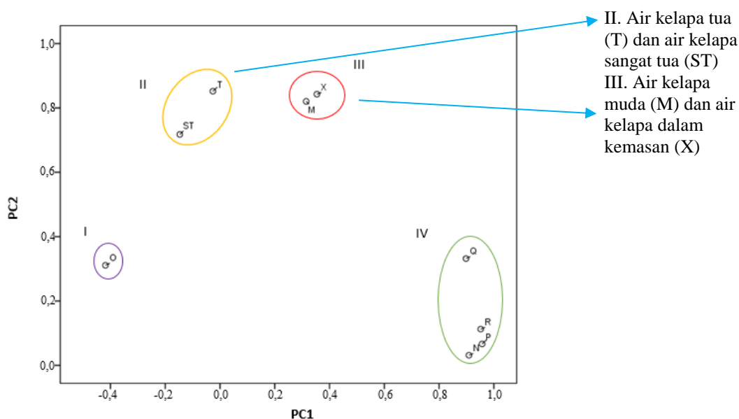
Gambar 3. Hasil PCA berdasarkan data derivatif pertama data absorbansi.
