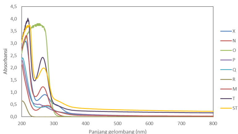
Gambar 1. Spektra UV-Vis dari 9 sampel yang dianalisis. M = Kelapa muda; T = Kelapa tua; ST = Kelapa sangat tua; N = Minuman isotonik 1; O = Minuman isotonik 2; P = Minuman isotonik 3; Q = Minuman isotonik 4; R = Air soda; X = Air kelapa dalam kemasan.
