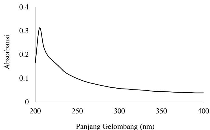
Gambar 4. Spektra Spektra absorbansi UV-Vis emulsi kosmetik 22% VCO
