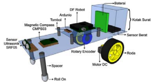
Gambar 7. Ilustrasi Robot Dengan Seluruh Komponen
