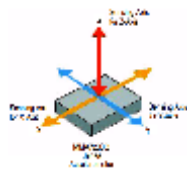
Gambar 1. Sumbu accelerometer
