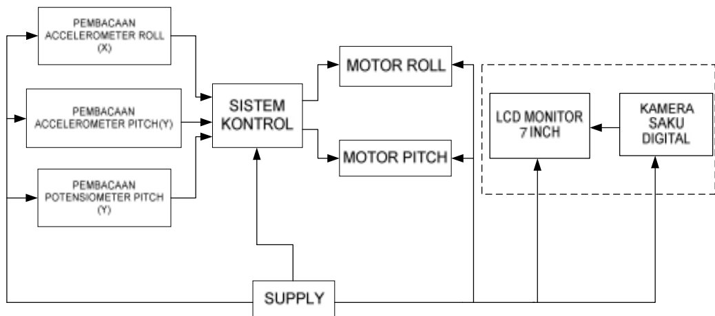
Gambar 2 Blok diagram sistem elektronik dan kendali
