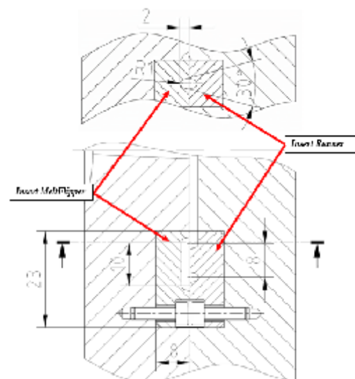
Gambar 10. Rancangan insert MeltFlipper dan insert runner
