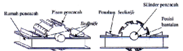
Gambar 12. Unit Pencacah Silinder Pencacah Tipe Reel
