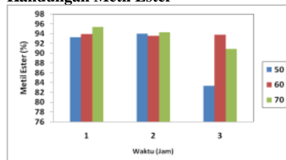
Gambar 2. Kandungan Metil Ester pada variasi konsentrasi 75 Gram KOH/100mL
