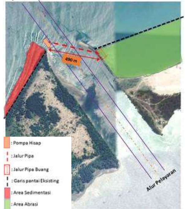
Gambar 4.4 Gambar Rencana perletakan pipa & pompa
