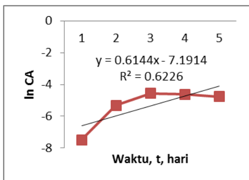
Gambar 4 Hubungan antara Waktu Maserasi dengan ln Ca
