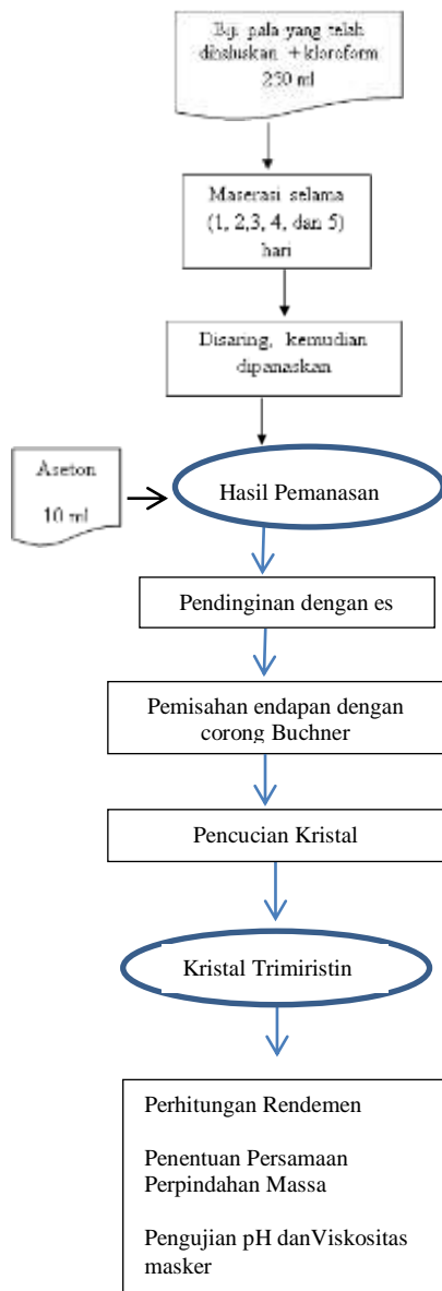
Gambar 1. Diagram alir Isolasi Trimiristin
