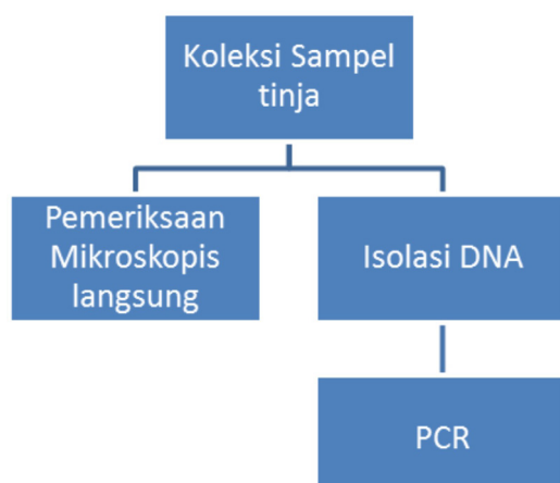
Gambar 1. Sistematika Penelitian
