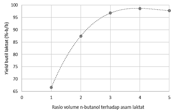
Gambar 6. Profil pengaruh rasio volume reaktan terhadap perolehan esterifikasi
