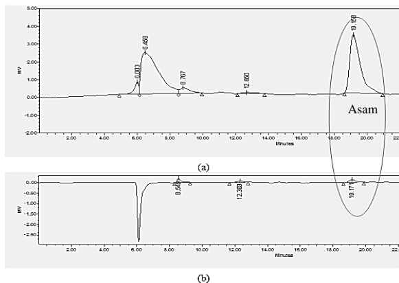
Gambar 9. Kromatogram produk fasa aquos (a) esterifikasi dan (b) hidrolisis
