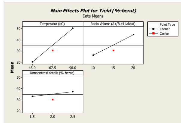
Gambar 3. Pengaruh variabel utama terhadap perolehan asam laktat pada reaksi hidrolisis
