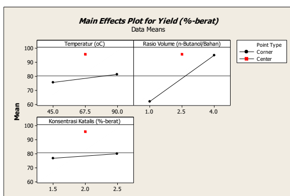
Gambar 2. Pengaruh variabel utama terhadap perolehan asam laktat pada reaksi esterifikasi
