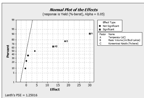
Gambar 5. Normal plot of the effects dari perolehan asam laktat pada reaksi hidrolisis
