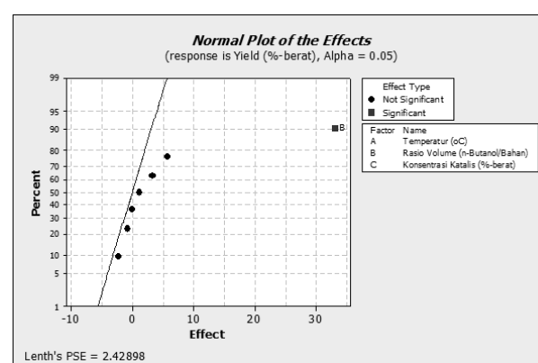
Gambar 4. Normal plot of the effects dari perolehan asam laktat pada reaksi esterifikasi
