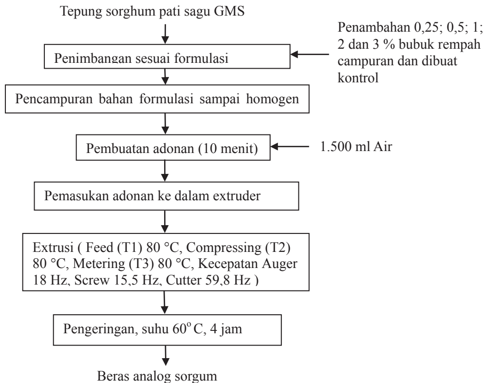
Gambar 1. Prosedur pembuatan beras analog (Budijanto dan Yuliyanti, 2012)
