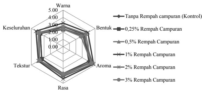
Gambar 4. Spider web hasil analisis karakteristik sensori nasi beras analog
