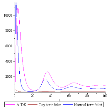
Gambar 4: Dinamika Perkembangan HIV/AIDS untuk 0 \leq t \leq 100
