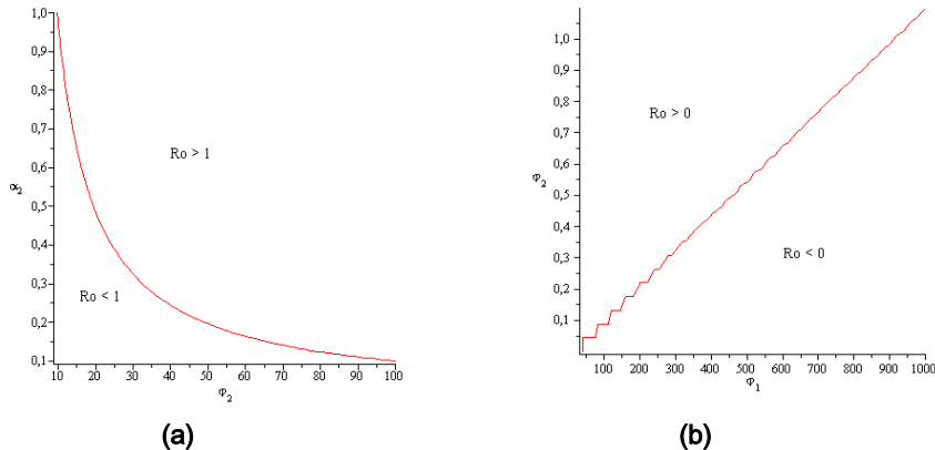
Gambar 2 : (a). Kurva dalam bidang \alpha_2 dan \varphi_2 , (b). Kurva dalam bidang \varphi_1 dan \varphi_2
