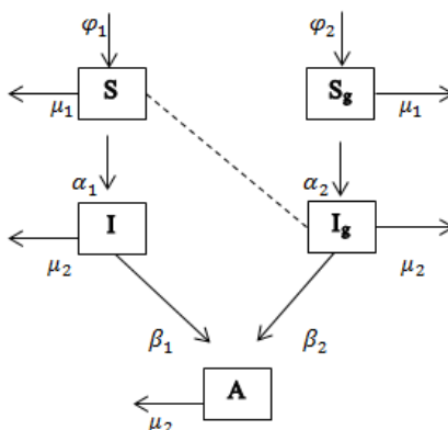
Gambar 1: Kompartemen Penyebaran HIV/AIDS
