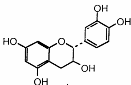
Gambar 1. Struktur Katekin
