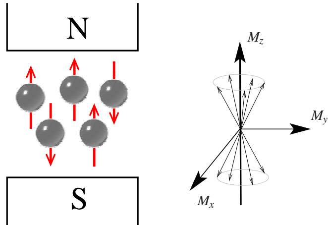
Figur 10: Disse figurer ses ofte, men er misvisende. De afspejler en fejlagtig opfattelse af, at spin kun kan være i spin-op eller i spin-ned tilstandene.
