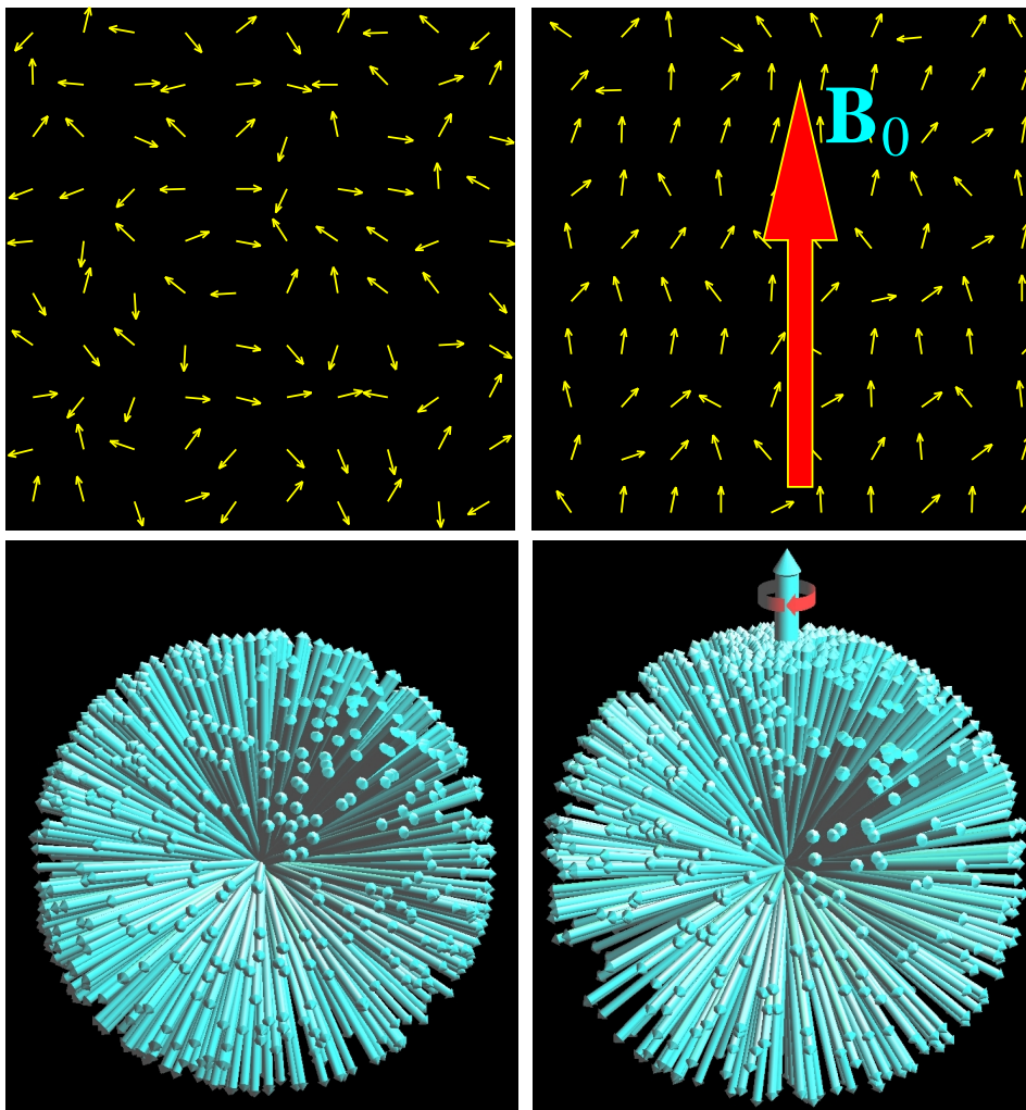
Figur 5: Figuren viser de samme situationer i to og tre dimensioner (øverst hhv. nederst). Kernespinne- nene er vist som talrige pile (vektorer). I de nederste grafer er de alle tegnet startende i samme punkt, således at fordelingen over retninger er tydelig (implicit koordinatsystem (M_x, M_y, M_z) ). Når patienten ankommer til afdelingen, er situationen, som vist i de to grafer til venstre: Spinnene er orienteret vilkårligt med en ensartet fordeling over retninger, dvs. omtrent lige mange spin peger i alle retninger. Nettomagnetiseringen er nær nul og kernerne præcesserer ikke. Når et magnetfelt \mathbf{B}_0 tilføjes, som vist i de to figurer til højre, opbygges en vis grad af ensretning (orden). Feltet er kun vist eksplicit i den øverste højre figur, men effekten er synlig i begge: Retningsfordelingen bliver "skæv" således at der er en overvægt af kerner pegende langs feltet. I nederste højre figur er både vist nettomagnetiseringen (tyk lodret pil) og præcessionen (kuglen roterer pga. magnetfeltet). De nederste figurer stammer fra artiklen Is Quantum Mechanics necessary for understanding Magnetic Resonance? Concepts in Magnetic Resonance Part A, 32A (5), 2008, http://www.drcmr.dk/MR .
