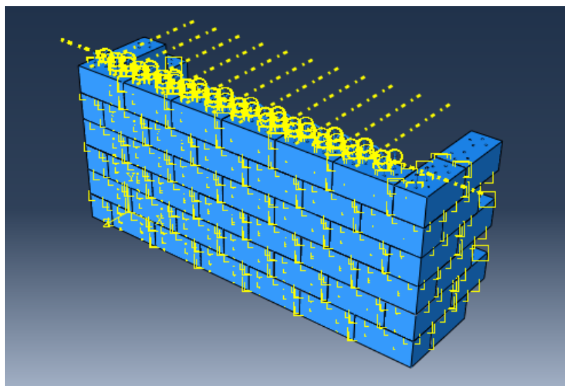
ILUSTRACIÓN 15.DETALLE DE LOS CONTACTOS EN EL MODELO
