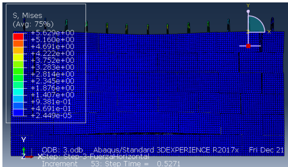
ILUSTRACIÓN 29. TENSIONES DE VON MISES
