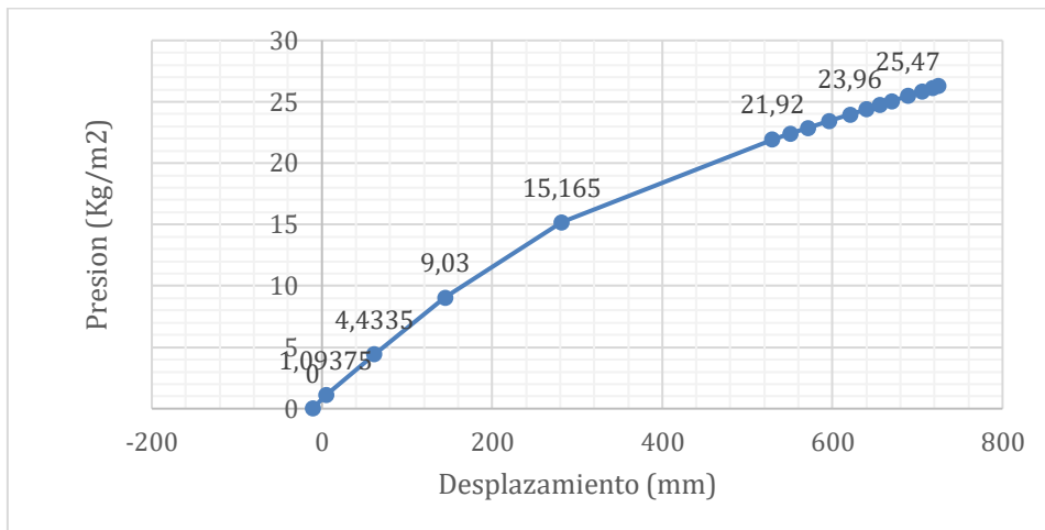
ILUSTRACIÓN 28. DESPLAZAMIENTO U3 FRENTE A LA CARGA DEL VIENTO APLICADA
