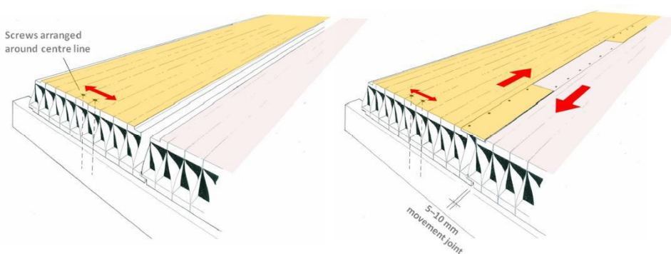
ILUSTRACIÓN 16.FORJADO KIELSTEG
