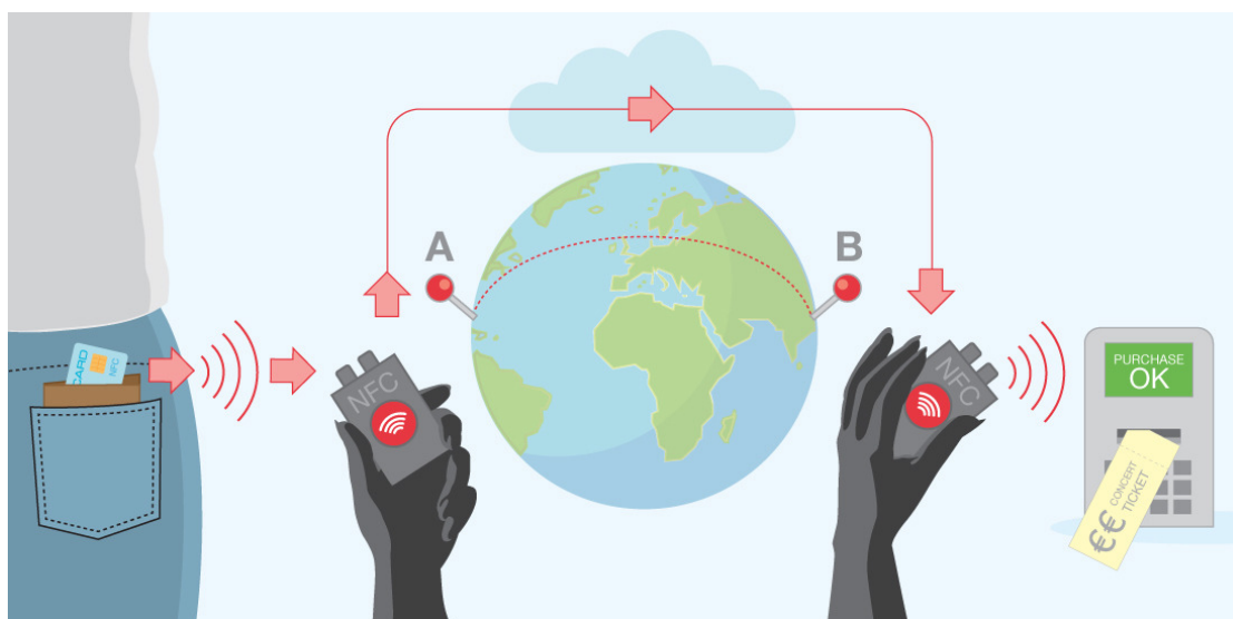
Figura 3.1: Ataque de retransmisión en sistemas de pago contactless , extraída de [22]
