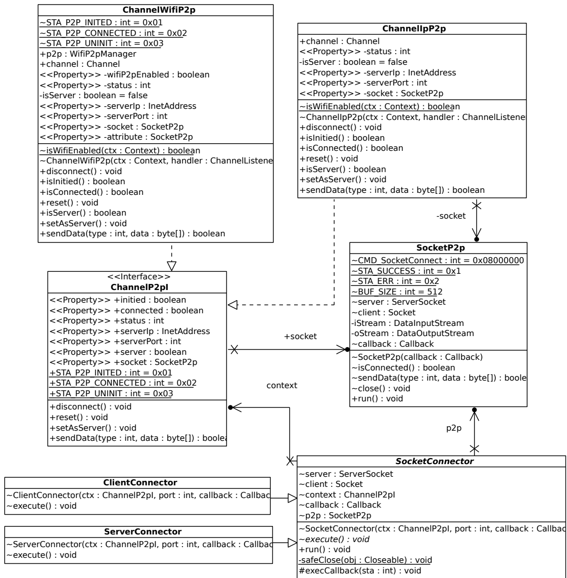
Figura 5.4: Diagrama de clases inicial para la implementación de la comunicación.
