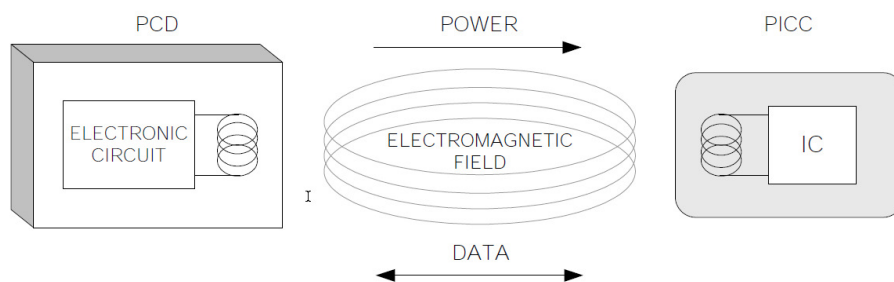
Figura 2.1: Configuración del PCD y PICC [9, página 13]
