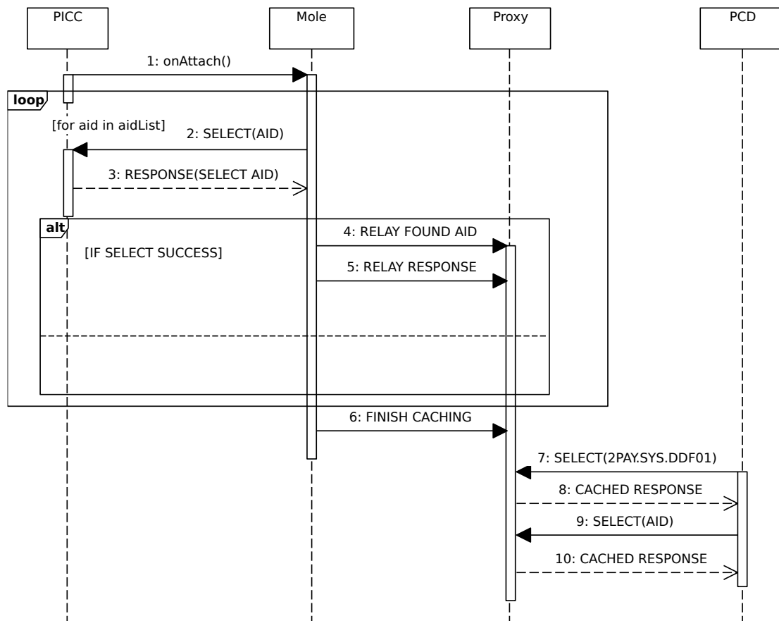
Figura 3.4: Diagrama de secuencia de la comunicación en un relay inteligente
