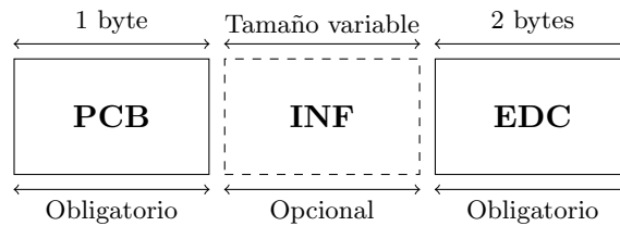
Figura 4.1: Bloque de transmisión de protocolo
