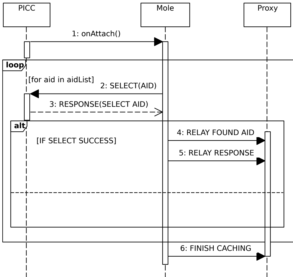
Figura 5.3: Diagrama de secuencia de la detección de AIDs y cacheado
