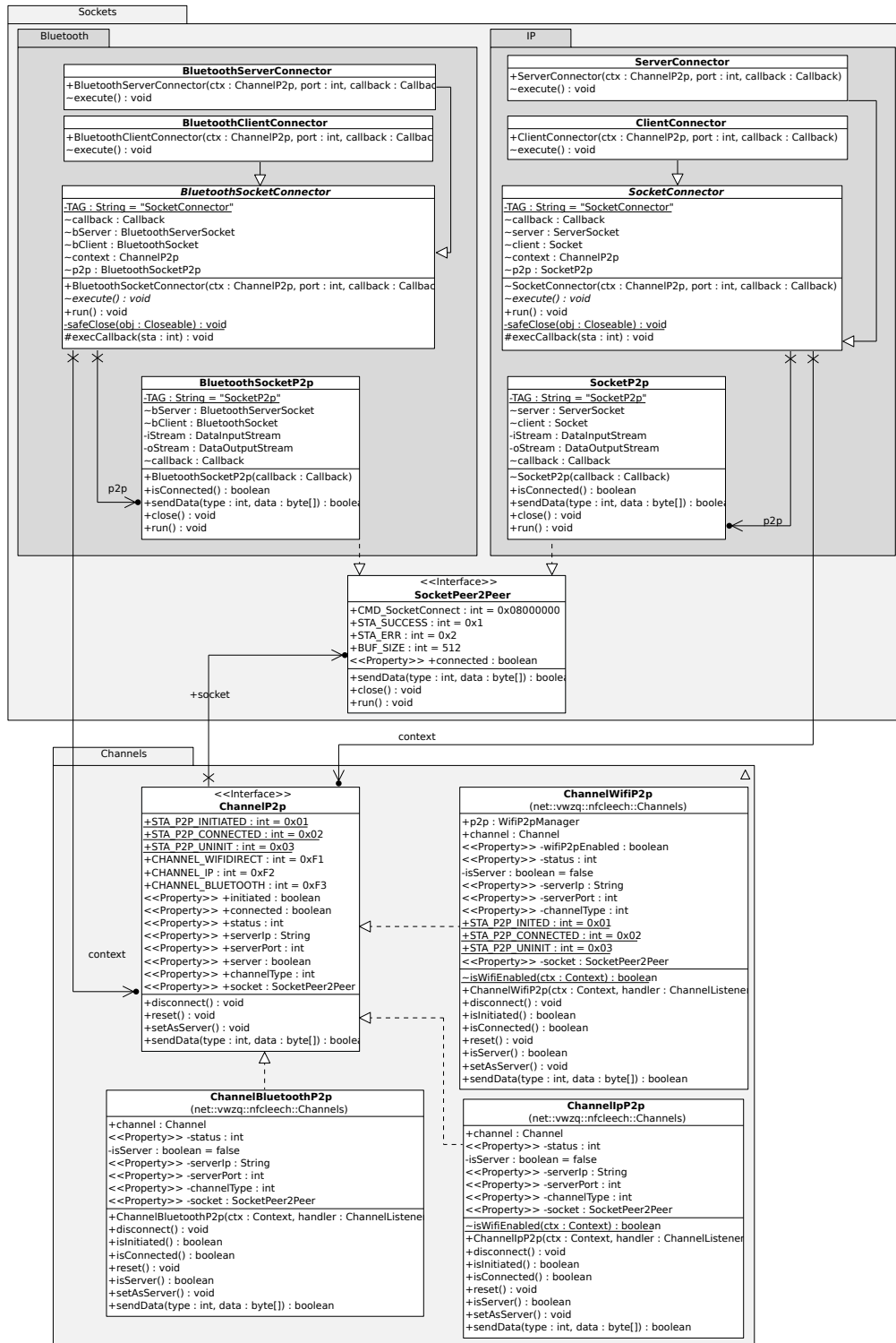
Figura 5.5: Diagrama de clases final para la implementación de la comunicación.
