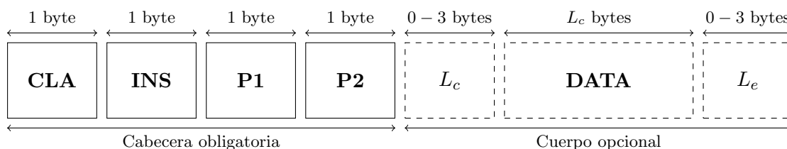
Figura 2.2: Comando APDU
