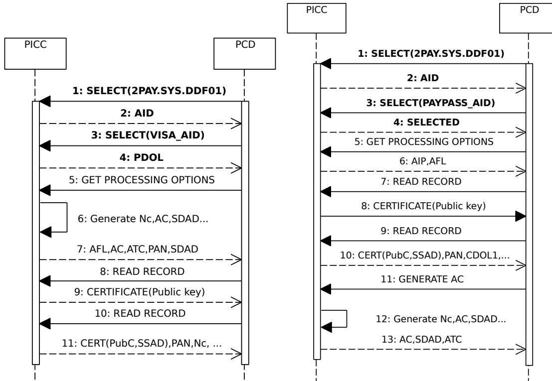
Figura 3.2: Diagrama de secuencia con Pay-Wave (VISA) [4]
