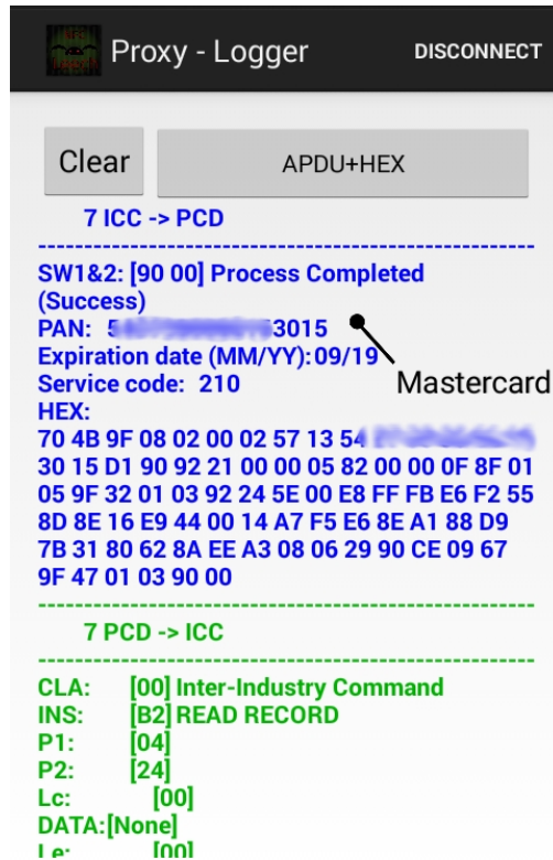
Figura 5.2: Ejemplo de interacción con MASTERCARD
