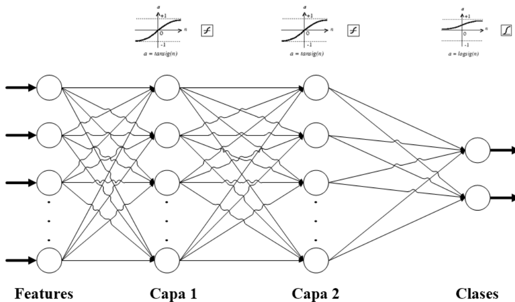
Fig. 24 Arquitectura MLP
