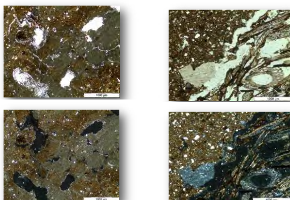
Figura 3: Paneles de microfotografías de los materiales edáficos en la actualidad. Calcificación (Izquierda) y Humificación (Derecha)
