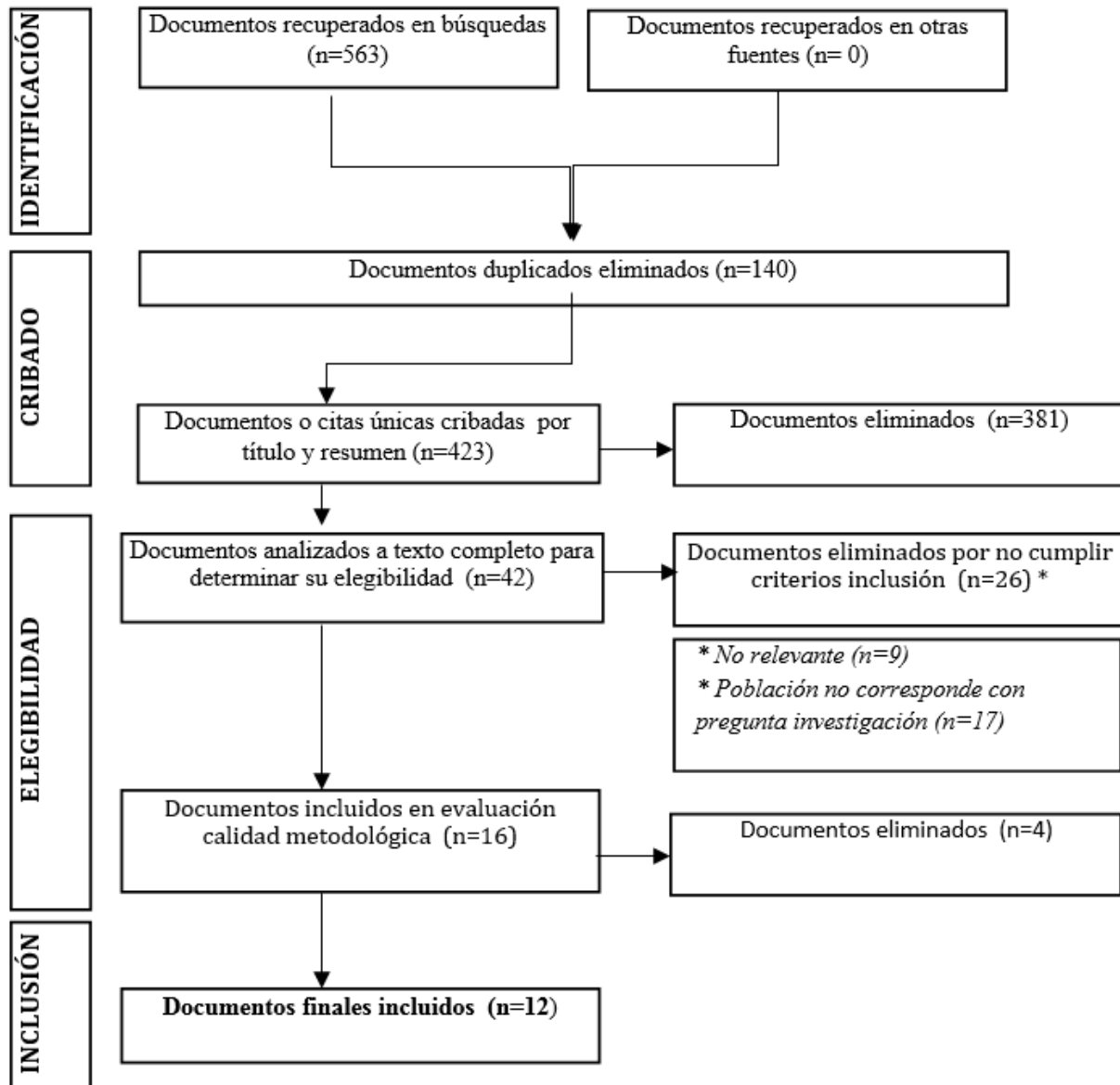
Figura 1. Flujograma PRISMA
