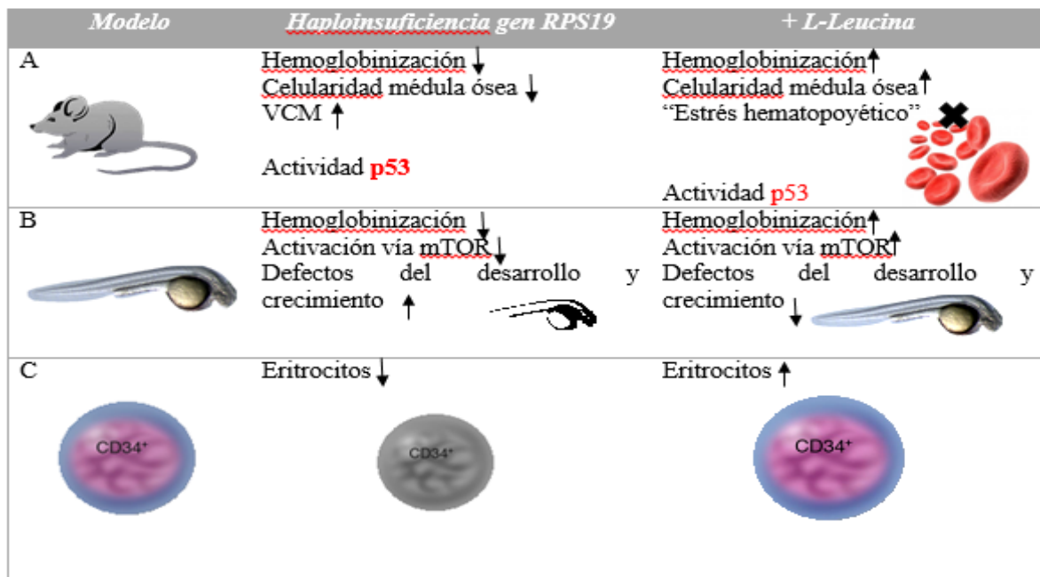
Figura 3. Objetivos clave encontrados en los tres principales sistemas estudiados donde se ha reproducido una haploinsuficiencia en el gen Rps19 23,21,24 . (A) El ratón inducido por doxiciclina descrito por Jaako et al 24 , mostró una reducción en la hemoglobinización e incremento del volumen corpuscular medio (VCM), con un decrecimiento en la celularidad de la médula ósea, y un evidente incremento en la actividad del p53. La administración de L-Leucina mostró una mejoría de estos síntomas, disminuyendo la actividad del p53, aumentando la hemoglobinización y celularidad de la médula ósea. (B) Payne et al 21 demostraron sobre el embrión de pez Zebra con haploinsuficiencia provocada por morfolino, también una disminución de la hemoglobinización, y en de la actividad de la vía mTOR, junto con un significativo aumento de defectos del desarrollo, los cuales fueron parcialmente aminorados con el tratamiento de L-Leucina. (C) La haploinsuficiencia provocada in vitro sobre las células humanas CD34+ realizado por Payne et al 21 , demostró una significativa disminución de la diferenciación en las células eritrocitarias. El tratamiento con L-Leucina incrementó el recuento eritrocitario. Ilustración adaptada de Marie Dauenheimer.
